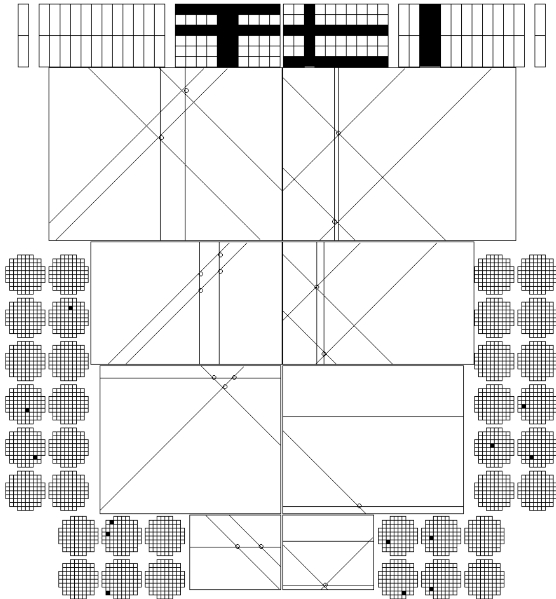
Abb. 2.7: Schematische Darstellung der Detektorsignale für ein Ereignis mit 4 Teilchen (nach Anwendung der Cluster-Erkennungs-Prozedur). Die Detektoren sind (von unten nach oben) innere Fasern, äußere Fasern, innere Drahtkammer, äußere Drahtkammern, Plastik-Hodoskop (innen), Cherenkov-Detektor (außen). Die karierten Kreise links und rechts stellen die Anoden der ortsauflösenden Photomultiplier dar, mit denen die Fasern ausgelesen werden. Die kleinen Kreise zeigen die Kombinationsmöglichkeiten innerhalb der Triplets, die nach der Dreifach-Koinzidenz-Suche noch erlaubt sind.
