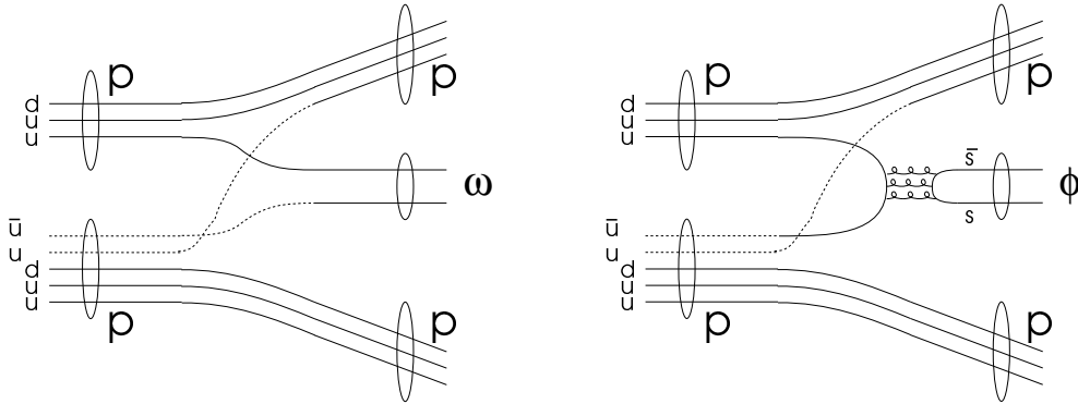
Abb. 1.2: Nach der OZI-Regel sind Prozesse, die nicht durch Diagramme mit zusammenhängenden Quark-Linien beschrieben werden können, stark unterdrückt. Unter der Annahme, daß \phi -Mesonen reine s\bar{s} -Zustände sind und Nukleonen keine s -Quarks enthalten, könnten \phi -Mesonen in pp -Stößen nur durch Diagramme höherer Ordnung mit dem Austausch von 3 Gluonen produziert werden.
