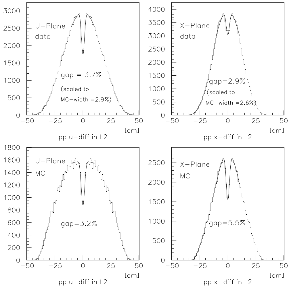
Abb. 4.7: Oben: Projektionen der Verteilung aus Abbildung 4.6 auf die U - und X -Koordinate. Unten: die entsprechenden Verteilungen für simulierte pp\phi Ereignisse. Die Prozentzahlen geben jeweils die relative Fläche des Minimums in der Mitte an. Zum besseren Vergleich sind oben zusätzlich auch die Werte angegeben, die man erhalten würde, wenn die Breite der Verteilung mit der aus der Simulation übereinstimmen würde.
