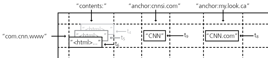
Abb. 21: Bigtable-Datenstruktur am Beispiel einer Webtable (Chang et al. 2006: 206)
