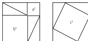
Abb. 33: Beweis des Satz des Pythagoras (Stjernfelt 2000: 369)
