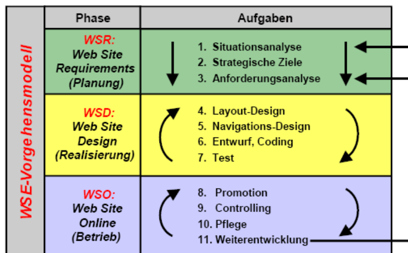
Abb. 12: Das WSE-Vorgehensmodell 113
