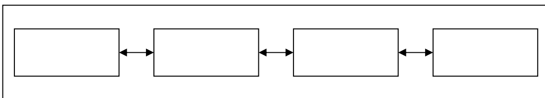
Abb. 7: Lineare Architektur
