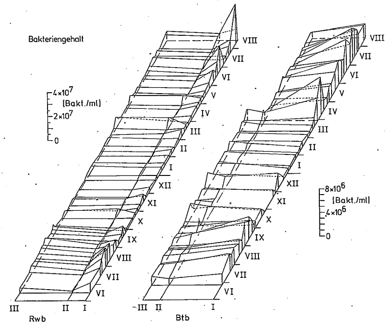
Abb. 1. Bakterienkonzentration (Bakterien auf Membranfiltern), Juni 1973 — August 1974. Die Zahlen an der Schmalseite geben die Untersuchungsstellen an, die an der breiten Seite die Monate. Die Lücken bei Rwb I (August 1973) und bei Btb I (November 1973) weisen auf die Austrocknung des Bachbettes an der jeweiligen Untersuchungsstelle hin. Zu beachten sind die unterschiedlichen Maßstäbe für Rohrwiesbach und Breitenbach.
