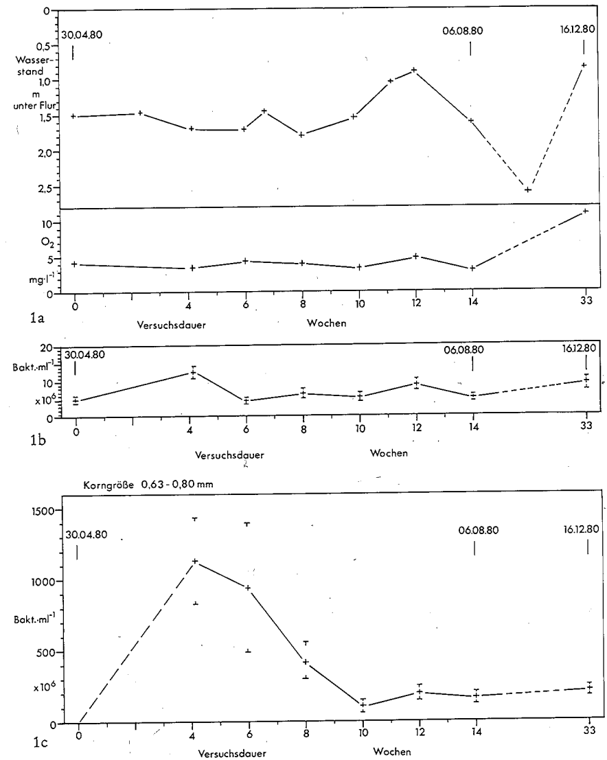
Abb. 1. Besiedlungsversuch 1980. a) (oben) Grundwasserstand und Sauerstoffgehalt im Grundwasser. b) (Mitte) Zahl der Bakterien im gepumpten Grundwasser, mit Vertrauensgrenzen der Zählungen (95 %). c) (unten) Zahl der Bakterien im Sediment, mit Vertrauensgrenzen (95 %). Die ersten Untersuchungen wurden 4 Wochen nach Beginn des Versuches durchgeführt. Daher wurde die Anfangsphase der Besiedlung nicht erfaßt.
