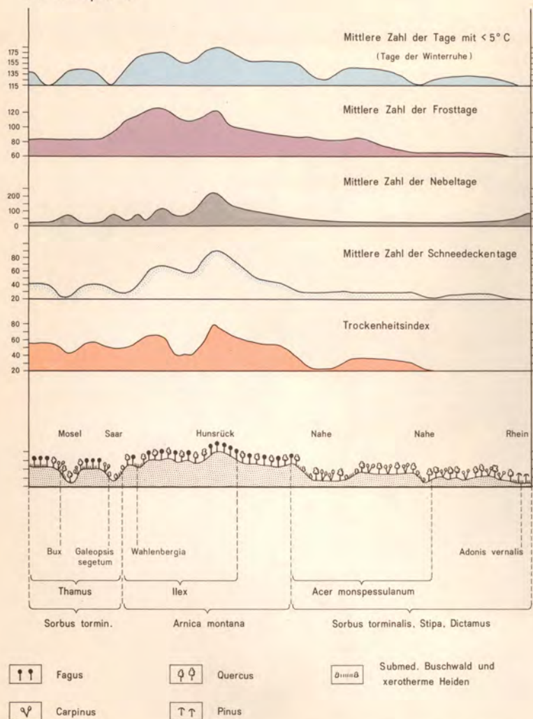
c) Klimaprofile
