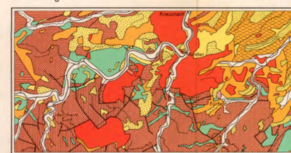
f) Geologie
