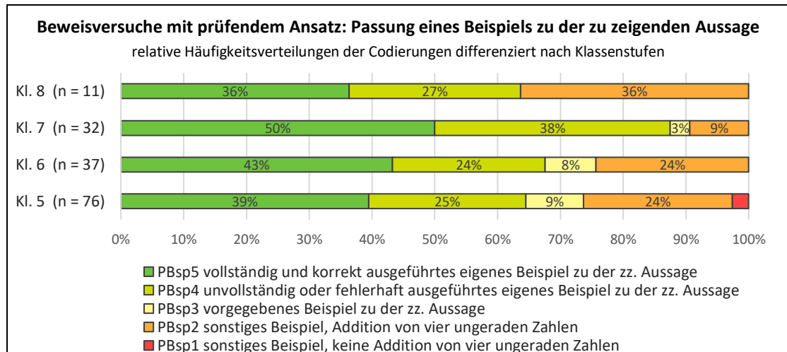
Abbildung 139: Beweisversuche mit prüfendem Ansatz: Passung eines Beispiels zu der zu zeigenden Aussage. Relative Häufigkeitsverteilungen der Codierungen differenziert nach Klassenstufen
