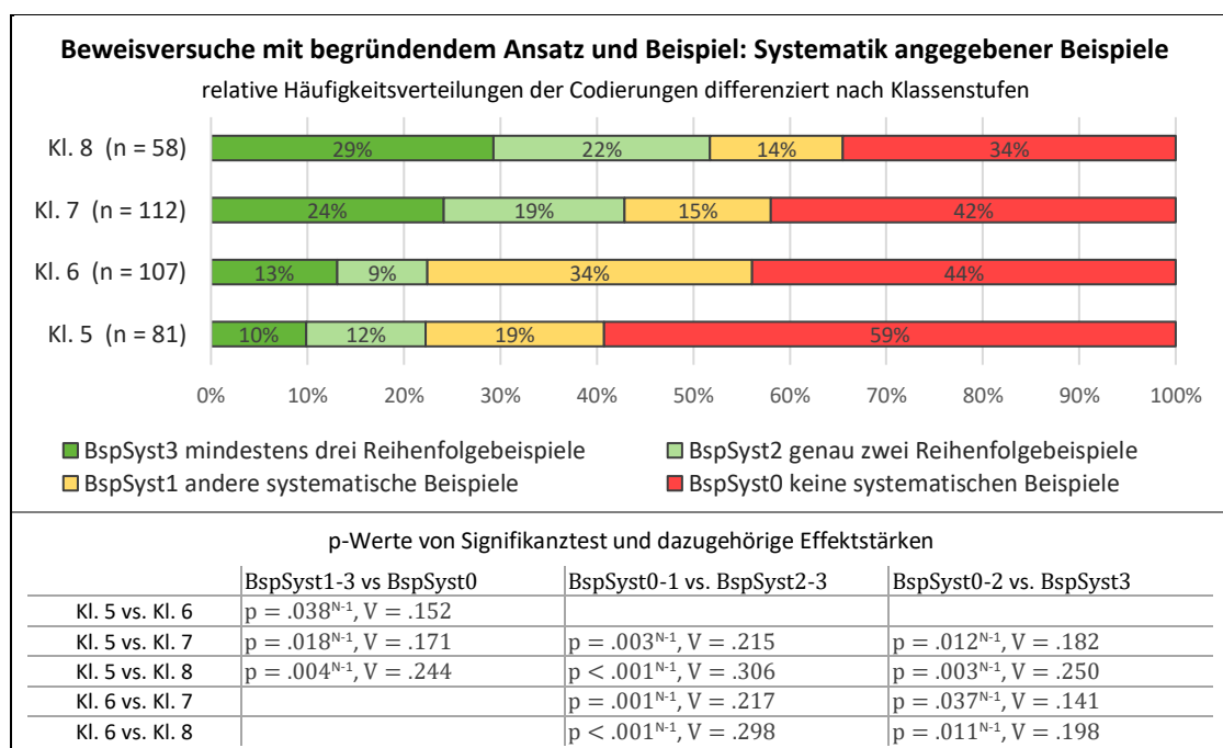
Abbildung 98: Beweisversuchen mit begründendem Ansatz und Beispiel: Systematik angegebener Beispiele. Relative Häufigkeitsverteilungen der Codierungen differenziert nach Klassenstufen sowie p-Werte von Signifikanztests, dazugehörige Effektstärken
