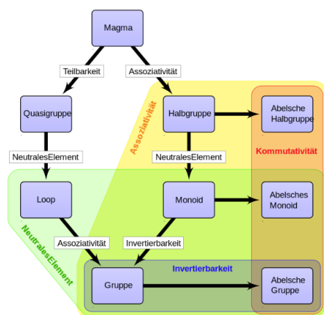
Abb. 37: Hierarchie algebraischer Strukturen (obere erfüllen weniger, untere mehr Gesetze) bis zur abelschen Gruppe.
