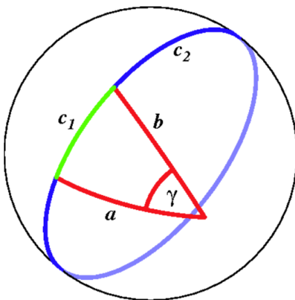
Abb. 43: Sphärisches Dreieck
