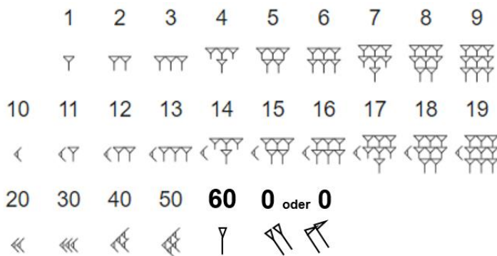
Abb. 25: Sumerische Zahlzeichen.
