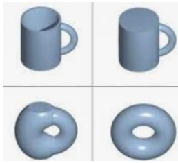
Abb. 39: Stetige Deformation
