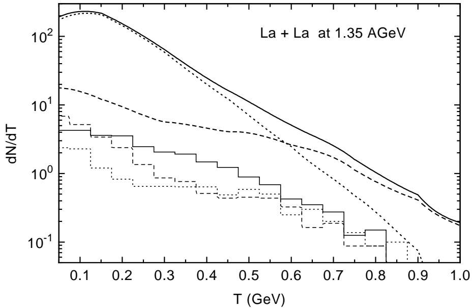
Abbildung 6.8: Pionenmultiplizität als Funktion der kinetischen Energie der Pionen im Schwerpunktsystem für eine zentrale ( b = 0 fm) La + La -Kollision bei einer Einschubenergie von 1.35 AGeV (durchgezogene Linie). Gepunktete Linie: Beiträge des \Delta(1232) -Zerfalls, der direkten Pionen-Produktion in Nukleon-Nukleon-Kollisionen und des Zerfalls der mesonischen Resonanzen \rho und \sigma zur Pionenmultiplizität. Gestrichelte Linie: Beiträge der höheren baryonischen Resonanzen. Die Beiträge einzelner baryonischer Resonanzen sind im unteren Teil der Abbildung durch Histogramme dargestellt: N(1440) durchgezogen, N(1535) gestrichelt und \Delta(1600) gepunktet.
