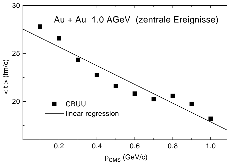
Abbildung 7.2: Mittlere Produktionszeit von Pionen für zentrale ( b = 0 \text{ fm} ) Au + Au -Reaktionen bei einer Einschussenergie von 1.0 \text{ AGeV} als Funktion des Pionenimpulses im Schwerpunktsystem der Reaktion. Die Vierecke geben die Ergebnisse des CBUU-Modells an und die durchgezogene Linie korrespondiert zu einem linearen Fit an diese Ergebnisse.
