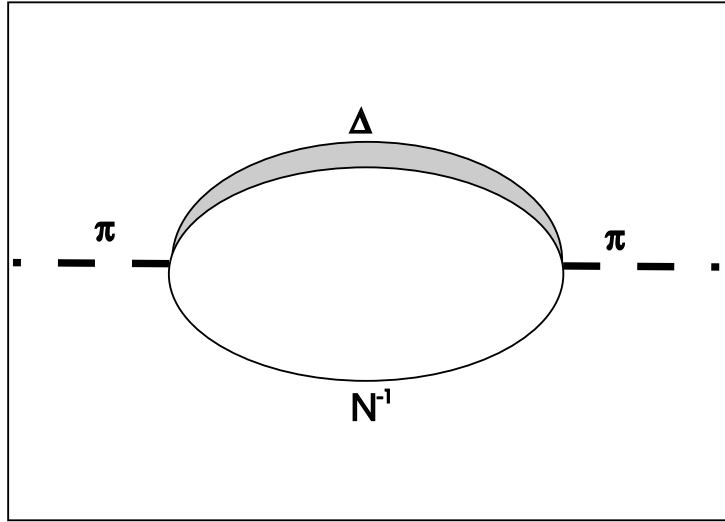
Abbildung 8.10: Polarisierungseinschub zur Bestimmung der Pionselbstenergie im Rahmen des \Delta -hole-Modells.
