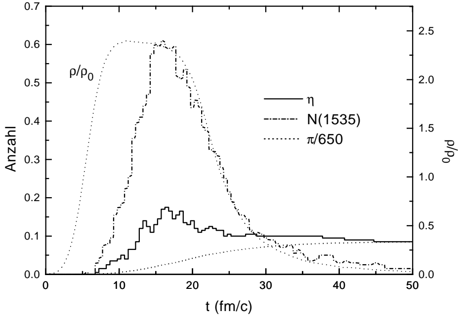
Abbildung 9.1: Zahl der in einer zentralen ( b = 0 fm) Au + Au -Kollision bei einer Einschussenergie von 1.0 AGeV vorhandenen \eta -Mesonen (durchgezogenes Histogramm), N(1535) (gestricheltes Histogramm) und Pionen skaliert mit 1/650 (strichpunktiertes Histogramm) als Funktion der Zeit. Die gepunktete Linie gibt die Baryondichte in Einheiten von \rho_0 im Zentrum der Reaktion an.
