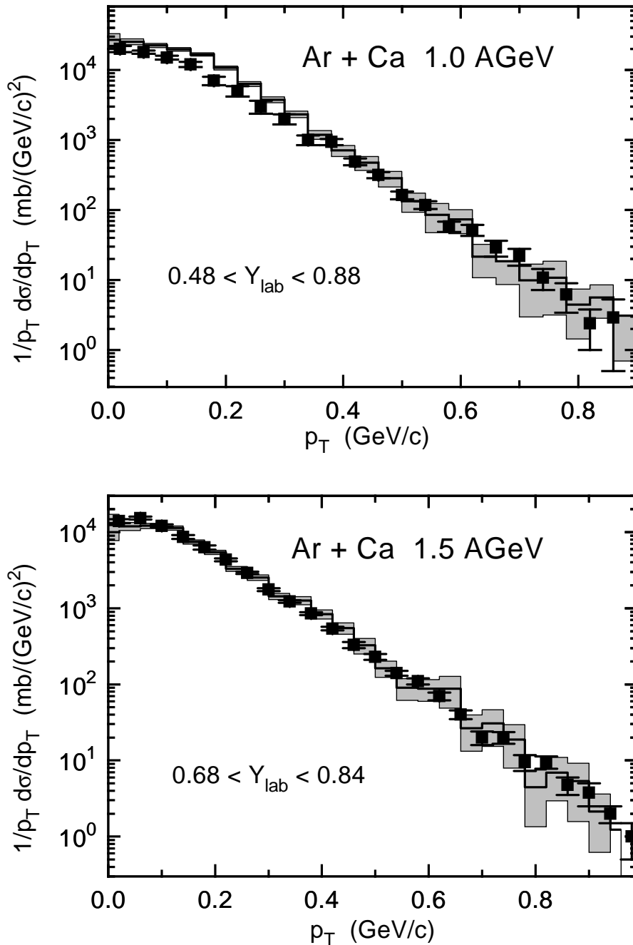
Abbildung 8.8: Wirkungsquerschnitt für die \pi^0 -Produktion in Ar + Ca -Kollisionen bei einer Einschußenergie von 1.0 (oben) und 1.5 (unten) AGeV für Labor-Rapiditäten von 0.48 \leq Y_{lab} \leq 0.88 bzw. 0.68 \leq Y_{lab} \leq 0.84 als Funktion des transversalen Impulses der Pionen. Die Ergebnisse der CBUU-Rechnungen werden durch die durchgezogenen Histogramme dargestellt. Die schraffierten Flächen geben die statistischen Fehler der Rechnungen an. Die experimentellen Daten der TAPS-Kollaboration [88, 89] sind durch die Vierecke dargestellt.
