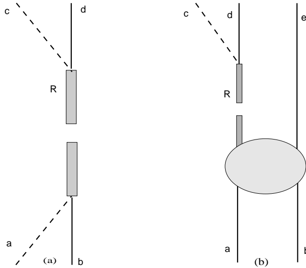
Abbildung 4.2: Meson-Nukleon (a) und Nukleon-Nukleon-Kollisionen (b) als Stufenprozesse im Resonanzmodell.
