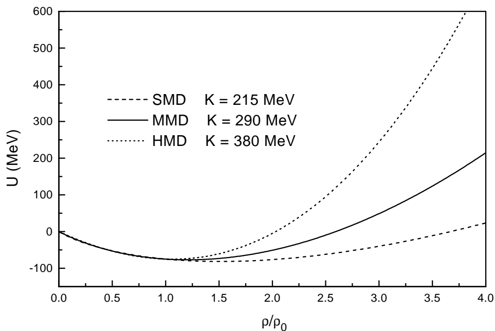
Abbildung 3.4: Resultierende Mittlere-Feld-Potentiale für die Parametersätze SMD , MMD und HMD (s. Tabelle (3.1)) für Nukleonen mit Impuls \vec{p} = \vec{0} .
