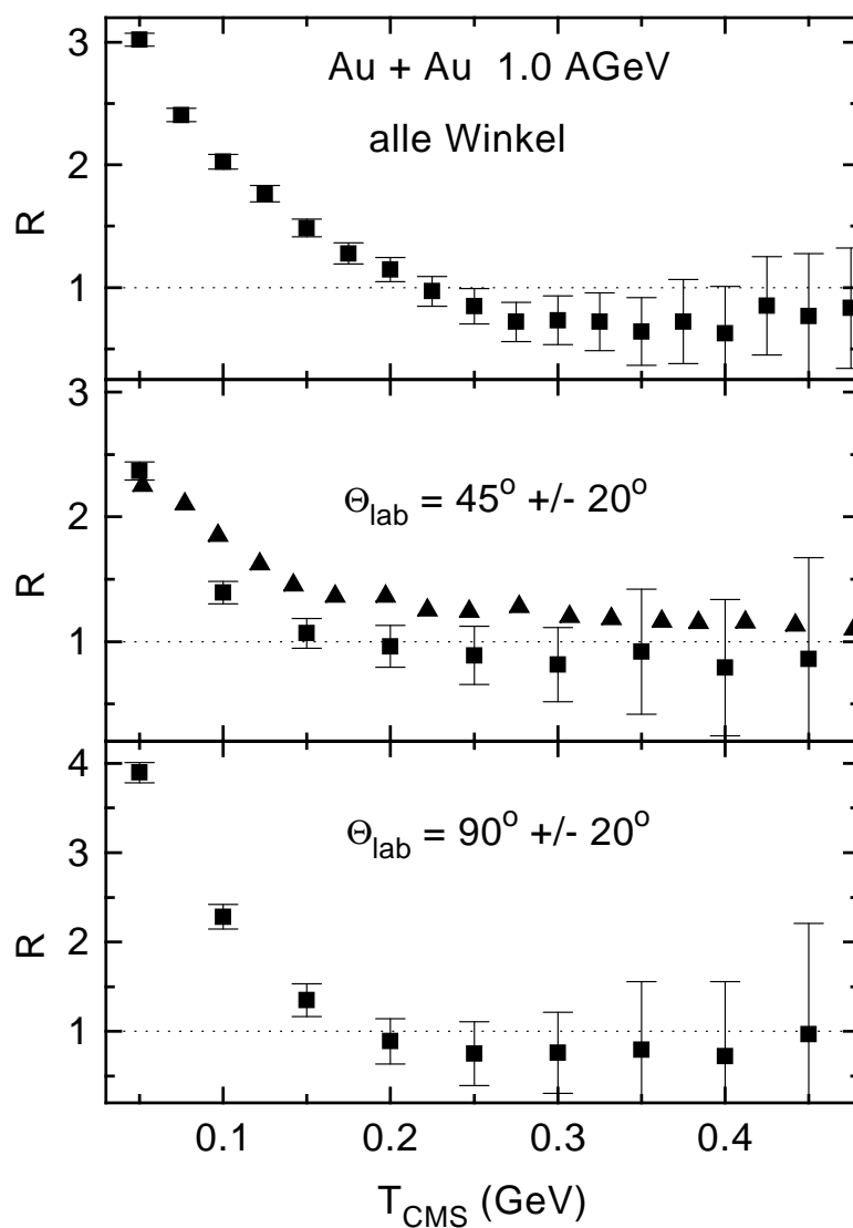
Abbildung 7.9: Das \pi^-/\pi^+ -Verhältnis für das System Au+Au bei einer Einschußenergie von 1.0 AGeV als Funktion der kinetischen Energie der Pionen im Schwerpunktsystem der Reaktion. Oben: R integriert über alle Winkel. Mitte: Für einen Laborwinkelbereich von 25^\circ \leq \Theta_{\text{lab}} \leq 65^\circ . Unten: Für einen Laborwinkelbereich von 70^\circ \leq \Theta_{\text{lab}} \leq 110^\circ . Die Fehlerbalken geben die statistischen Fehler der Rechnung an. Die Dreiecke im mittleren Teil der Abbildung geben die experimentellen Daten der KaoS-Kollaboration für 40^\circ \leq \Theta_{\text{lab}} \leq 48^\circ [83] an.
