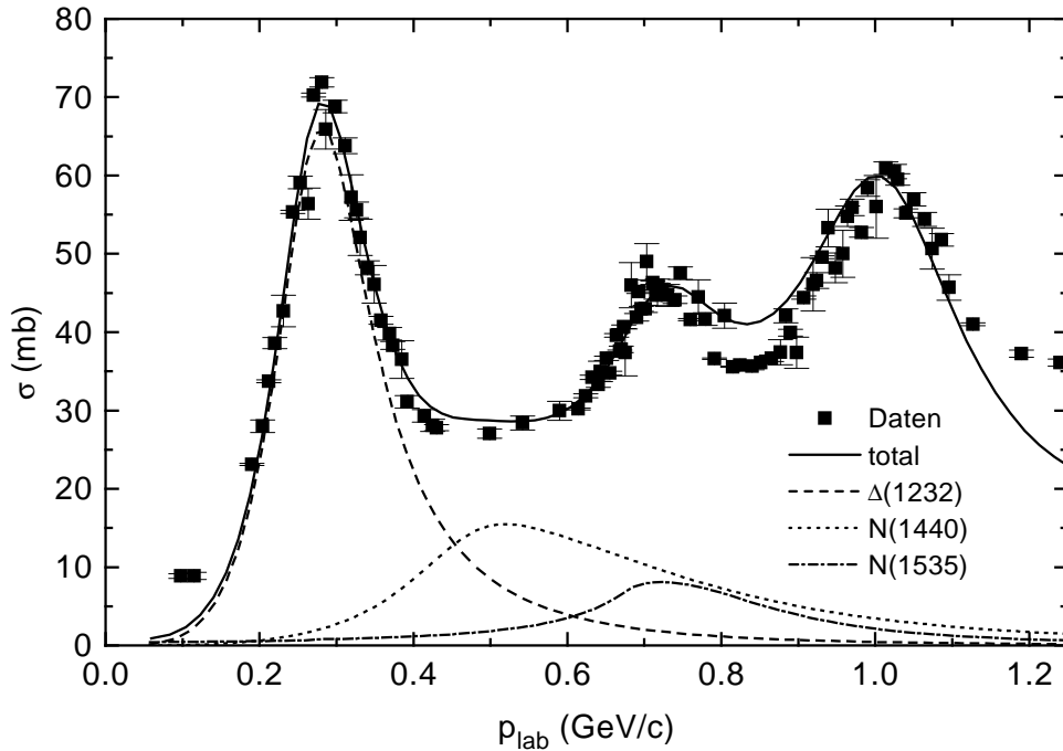
Abbildung 4.3: Der totale Wirkungsquerschnitt der Reaktion \pi^-p in Breit-Wigner-Näherung als Funktion des \pi -Laborimpulses ( durchgezogene Linie) im Vergleich zu den experimentellen Daten [68]. Die gestrichelte, die gepunktete und die strich-punktete Linie geben die Beiträge des \Delta(1232) , des N(1440) und des N(1535) zum totalen Wirkungsquerschnitt an.
