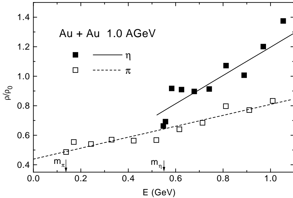
Abbildung 9.2: Die mittlere Ausfrierdichte der \eta - (ausgefüllte Vierecke) und \pi -Mesonen (offene Vierecke) einer Au + Au -Kollision bei einer Einschussenergie von 1.0 \text{ AGeV} als Funktion der Energie im Schwerpunktsystem der Reaktion. Die Linien korrespondieren zu linearen Fits an die CBUU-Resultate. Es wurden Ereignisse mit Stoßparametern im Bereich zwischen 0 und 16 \text{ fm} berücksichtigt.
