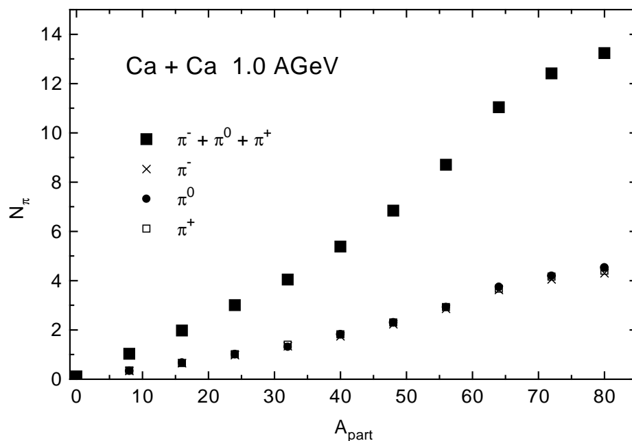
Abbildung 6.16: Zahl der in Ca + Ca -Kollisionen bei einer Einschubenergie von 1.0 AGeV produzierten Pionen (Vierecke) als Funktion von A_{part} . Die Zahl der produzierten \pi^+ , \pi^0 und \pi^- werden durch die offenen Vierecke, die Punkte bzw. die Kreuze dargestellt, die wegen der Isospinsymmetrie des Systems alle zusammenfallen. Die statistischen Fehler der Rechnung sind kleiner als die zur Darstellung verwendeten Symbole.
