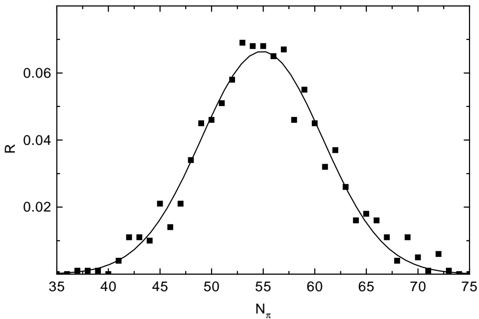
Abbildung 6.18: Relative Anzahl R der CBUU-Ereignisse einer Au + Au -Kollision bei einer Einschußenergie von 1.0 AGeV und einem Stoßparameter von 0 fm als Funktion der produzierten Pionen (Vierecke). Die durchgezogene Linie repräsentiert eine Gauß-Interpolation an die CBUU-Ergebnisse.
