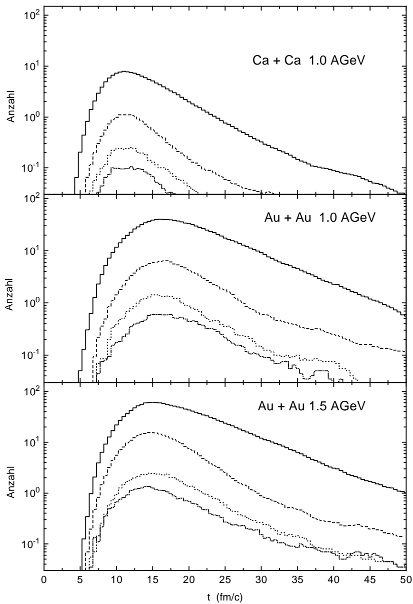
Abbildung 6.2: Die Zahl der \Delta(1232) (durchgezogene Histogramme), die Summe der höheren baryonischen Resonanzen (gestrichelte Histogramme), die Zahl N(1440) (gepunktete Histogramme) und die Zahl der N(1535) (strichpunktierte Histogramme) für zentrale ( b = 0 fm) Kollisionen als Funktion der Zeit. Oben: Ca + Ca bei 1.0 AGeV, Mitte: Au + Au bei 1.0 AGeV und unten: Au + Au bei 1.5 AGeV.
