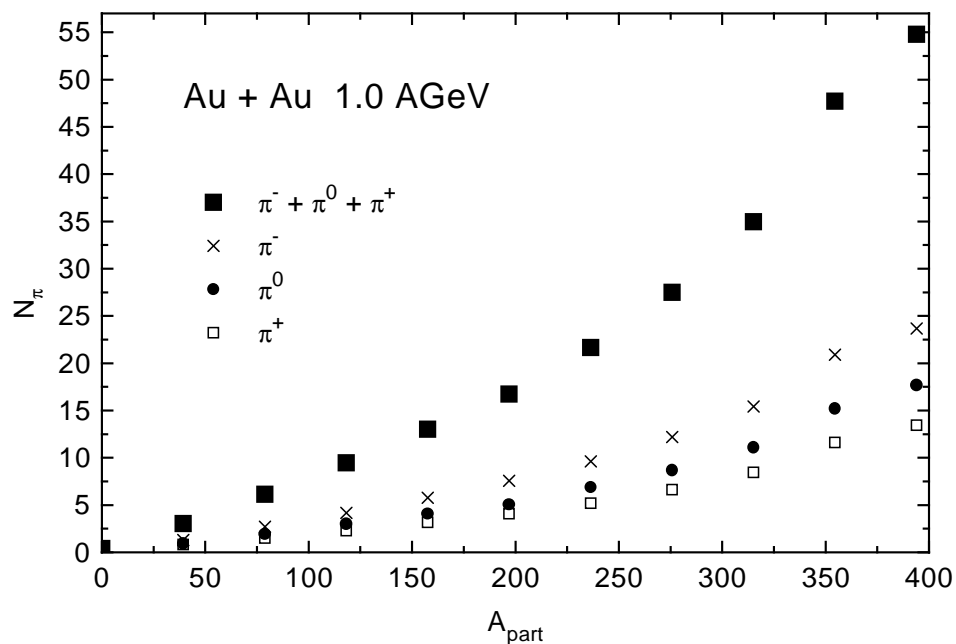
Abbildung 6.15: Zahl der in Au + Au -Kollisionen bei einer Einschubenergie von 1.0 AGeV produzierten Pionen (Vierecke) als Funktion von A_{part} . Die Zahl der produzierten \pi^+ , \pi^0 und \pi^- werden durch die nach unten bzw. nach oben gerichteten Dreiecke und die Kreise dargestellt. Die statistischen Fehler der Rechnung sind kleiner als die zur Darstellung verwendeten Symbole.
