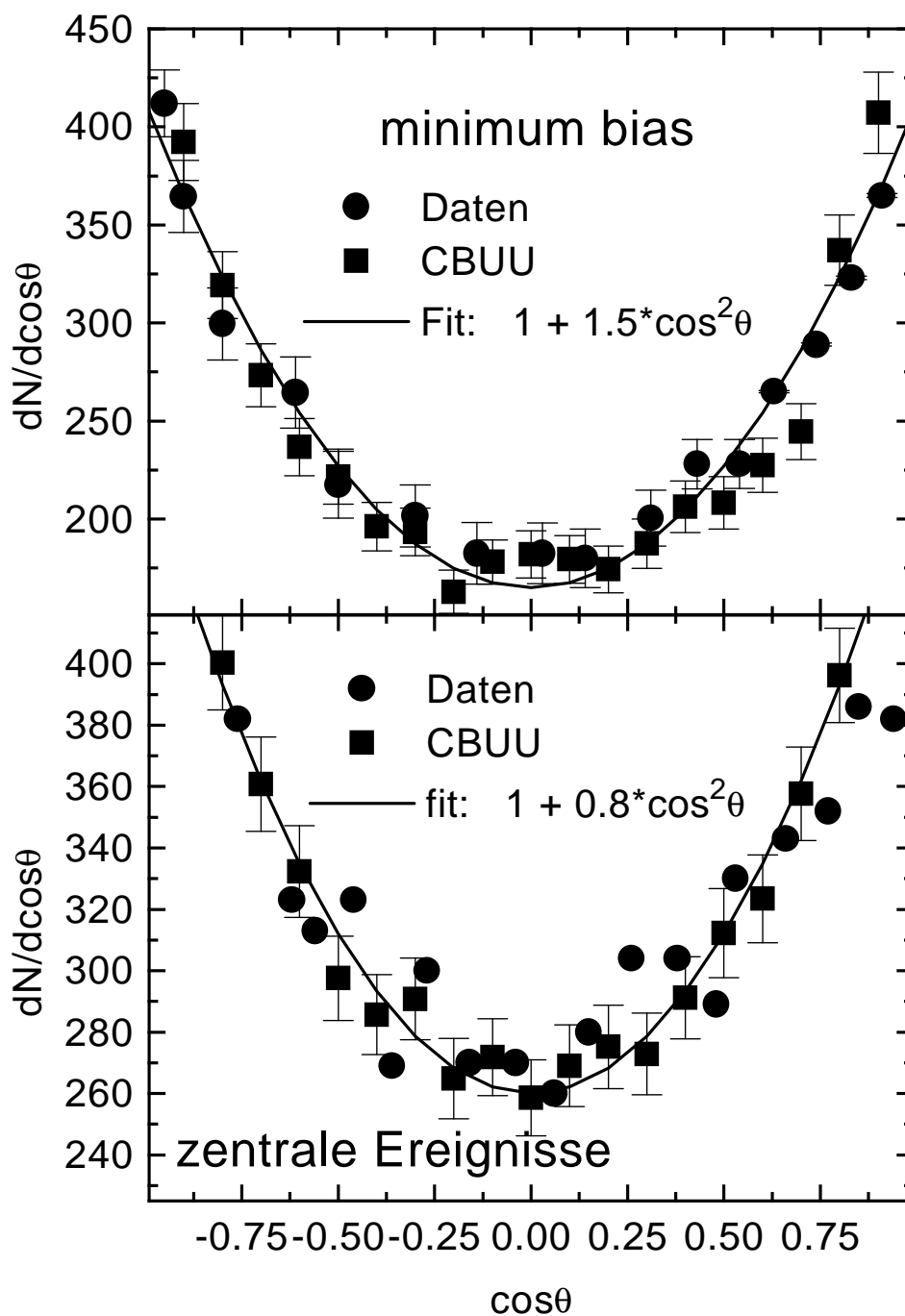
Abbildung 8.4: Zahl der \pi^- -Mesonen als Funktion von \cos\Theta_{CMS} für 'minimum bias' (oben) und zentrale (unten) Ereignisse im Schwerpunktsystem der Reaktion. Die experimentellen Daten aus [85] werden durch die Kreise und die Ergebnisse der CBUU-Rechnung durch die Vierecke dargestellt. Die durchgezogenen Linien korrespondieren zu Fits der Form (8.2) an die CBUU-Rechnungen.
