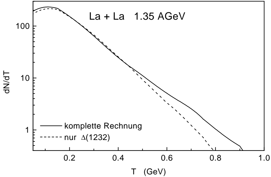
Abbildung 6.7: Pionenmultiplizität als Funktion der kinetischen Energie der Pionen im Schwerpunktsystem für eine zentrale ( b = 0 fm) La + La -Kollision bei einer Einschussenergie von 1.35 AGeV. Die durchgezogene Linie korrespondiert zu einer Rechnung im Rahmen des CBUU-Modells. Die gestrichelte Linie repräsentiert das Ergebnis einer Rechnung ohne höhere baryonische Resonanzen.
