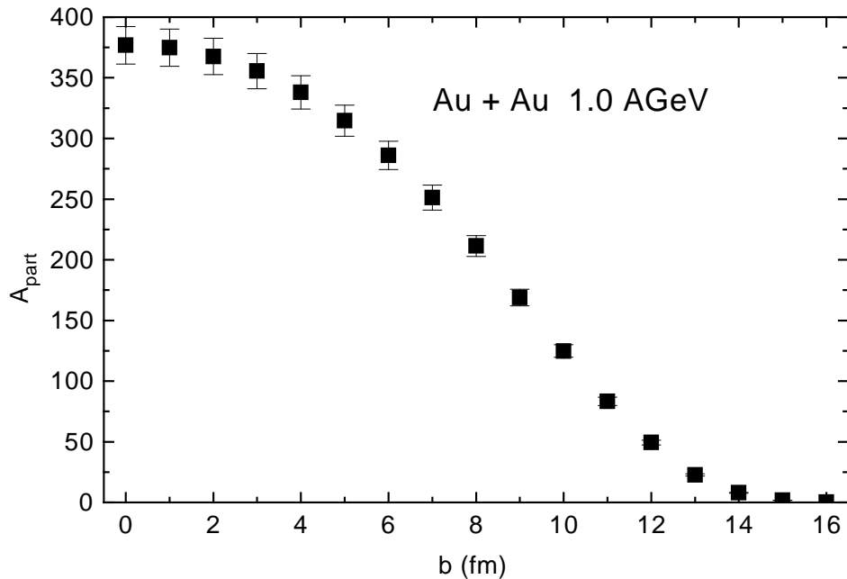
Abbildung 6.14: Zahl der Nukleonen A_{part} , die an mindestens einer elementaren Baryon-Baryon-Kollision teilgenommen haben, als Funktion des Stoßparameters. A_{part} ist für die Reaktion Au + Au bei einer Einschußenergie von 1.0 AGeV dargestellt. Die Fehlerbalken geben die statistischen Fehler der Rechnung an.
