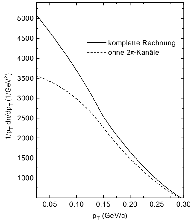
Abbildung 6.10: Totale Pionenmultiplizität gewichtet mit 1/p_T für eine zentrale Au+Au Kollision bei einer Einschußenergie von 1.5 AGeV. Die durchgezogene Linie stellt das Ergebnis einer kompletten CBUU-Rechnung dar und die gestrichelte Linie wurde unter Vernachlässigung der 2\pi -Kanäle (s. Text) erhalten.
