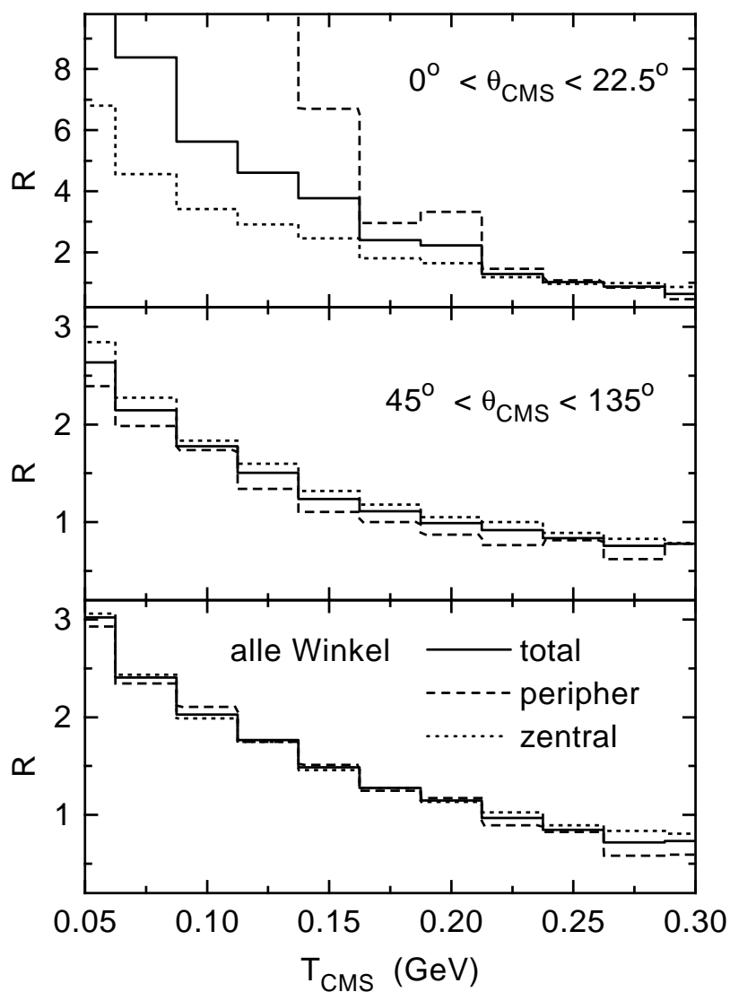
Abbildung 7.8: Das Verhältnis R für die Reaktion Au+Au bei einer Einschubenergie von 1.0 AGeV für alle (durchgezogene Histogramme), periphere ( 6 < b \leq 16 fm, gestrichelte Histogramme) und zentrale ( 0 \leq b \leq 6 fm, gepunktete Histogramme) Ereignisse als Funktion der kinetischen Energie der Pionen im CMS. Oben: Für Pionen, die unter \Theta_{CMS} = 0^\circ \pm 22.5^\circ emittiert werden. Mitte: Für Pionen, die die Reaktionszone in einem Winkelbereich von 45^\circ \leq \Theta_{CMS} \leq 135^\circ verlassen. Unten: Integriert über alle Winkel.
