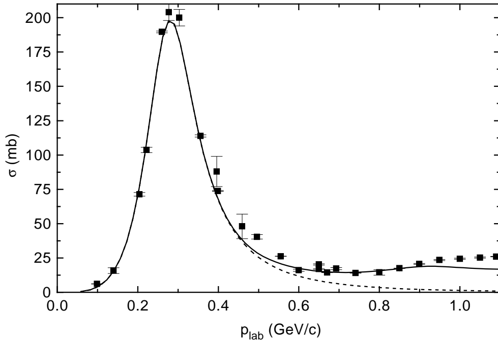
Abbildung 4.4: Der totale Wirkungsquerschnitt der Reaktion \pi^+p aus Gleichung (4.15) als Funktion des \pi -Laborimpulses ( durchgezogene Linie) im Vergleich zu den experimentellen Daten [68]. Die gestrichelte Linie gibt den Beitrag des \Delta(1232) zum totalen Wirkungsquerschnitt an.
