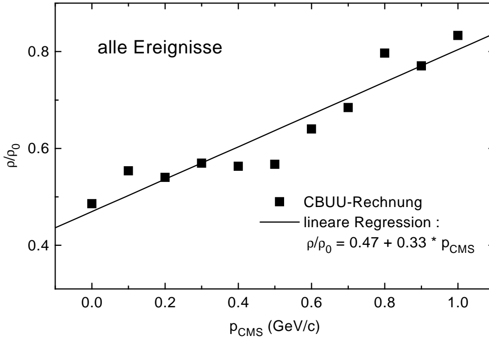
Abbildung 7.3: Mittlere Baryonendichte am Produktionsort der Pionen für die Reaktion Au + Au bei einer Einschubenergie von 1.0 AGeV als Funktion des Pionenimpulses im Schwerpunktsystem der Reaktion. Die Vierecke geben die Ergebnisse des CBUU-Modells an und die durchgezogene Linie korrespondiert zu einem linearen Fit an diese Ergebnisse.
