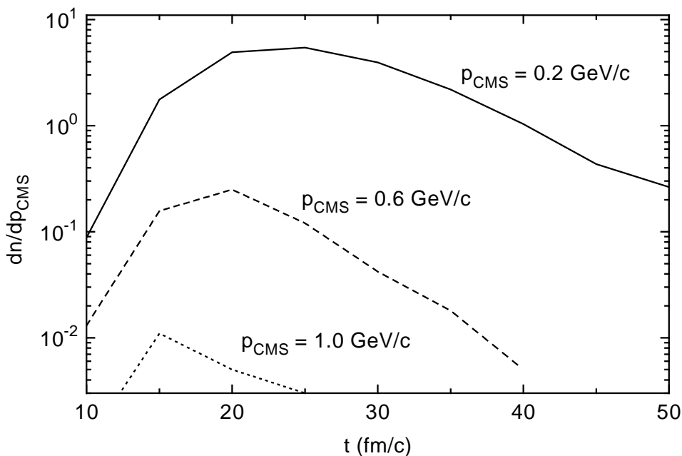
Abbildung 7.1: Zahl der am Ende der Reaktion Au + Au bei 1.0 \text{ AGeV} beobachteten Pionen als Funktion ihrer Produktionszeit für drei verschiedene kinematische Bereiche. Es wurden nur zentrale Ereignisse ( b = 0 \text{ fm} ) berücksichtigt. Die durchgezogene Linie korrespondiert zu Impulsen von 0.2 \text{ GeV}/c , die gestrichelte Linie zu Impulsen von 0.6 \text{ GeV}/c und die gepunktete Linie zu Impulsen von 1.0 \text{ GeV}/c im Schwerpunktsystem der Schwerionenreaktion.
