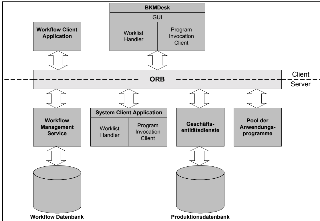
Abb. 4: Systemarchitektur der „Neuen Kernanwendung“ der BKM (vereinfacht) 32
