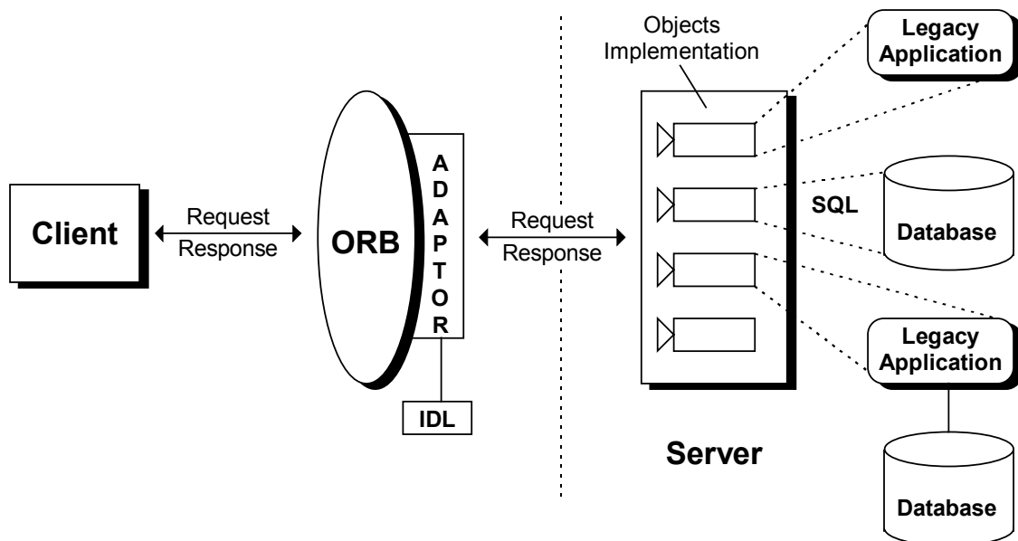
Abb. 1: Funktionsweise der Client/Server-Struktur in CORBA 14
