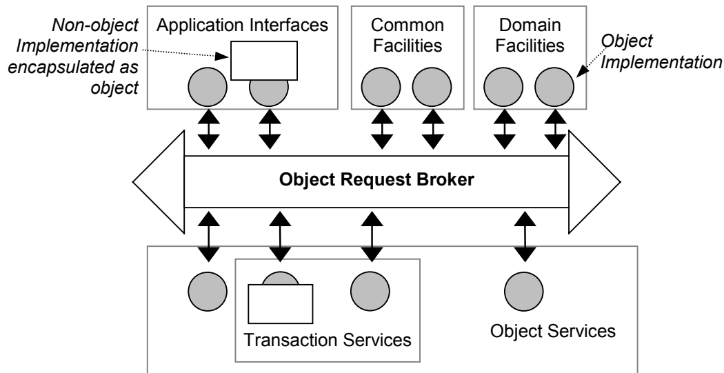
Abb. 2: Architektur für das Management verteilter Objekte 15
